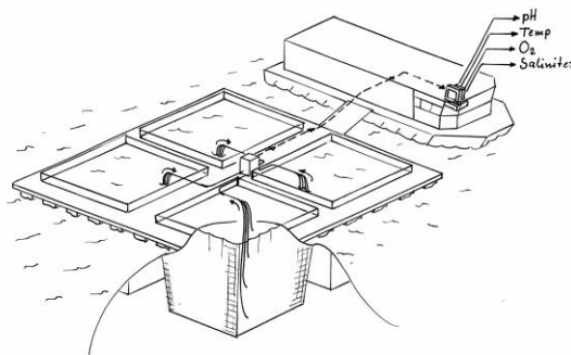
Figur 1. Måleprinsipp, vannkvalitetsrobot
